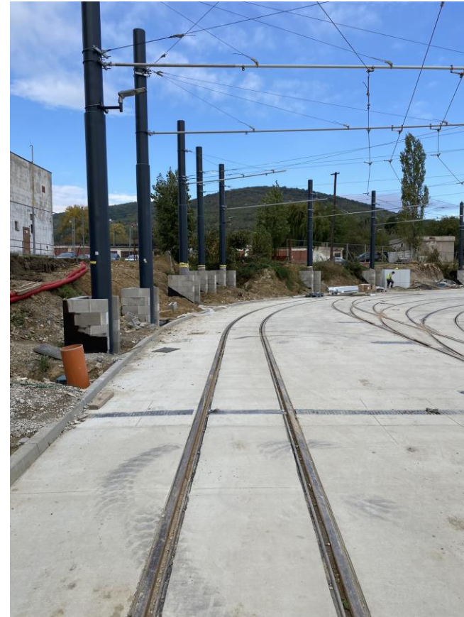
Obr. 11 – Dokončený koľajový zvršok
